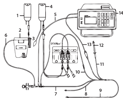
1. attēls. Noslēgtas sistēmas uzstādīšana
