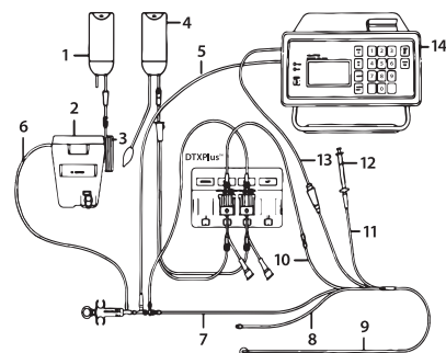
Rysunek 1. Konfiguracja systemu zamkniętego obiegu
