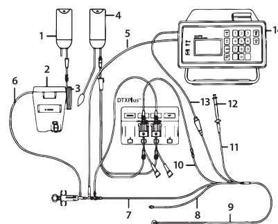
Фигура 1. Настройване на система със затворен цикъл
