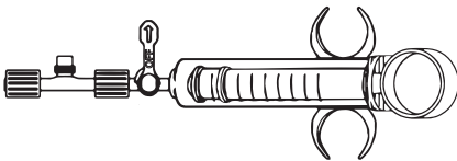
Afbeelding 2. Sensorbehuizing, afsluitkraan en spuit
