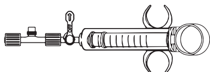
Figura 2. Compartimento do sensor, torneira e seringa
