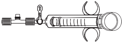
Figura 2. Alojamento do sensor, válvula reguladora e seringa
