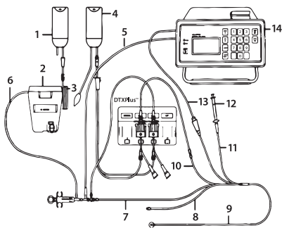
Şekil 1. Kapalı Döngü Sistemi Kurulumu
