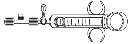
Şekil 2. Sensör Yuvası, Vana ve Şırınga
