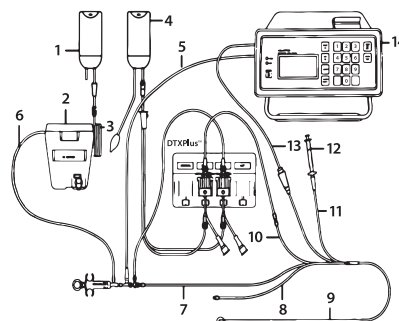
Εικόνα 1. Ρύθμιση συστήματος κλειστού βρόχου
